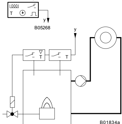
Газовый котел с атмосферной горелкой
